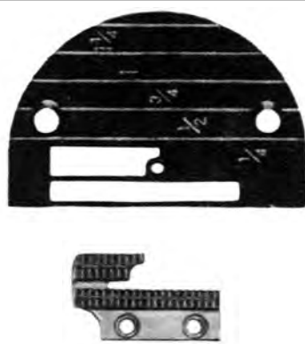
placca 26605LG griffa 26603 (149603)
