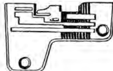
204867-0-10 Needle plate
